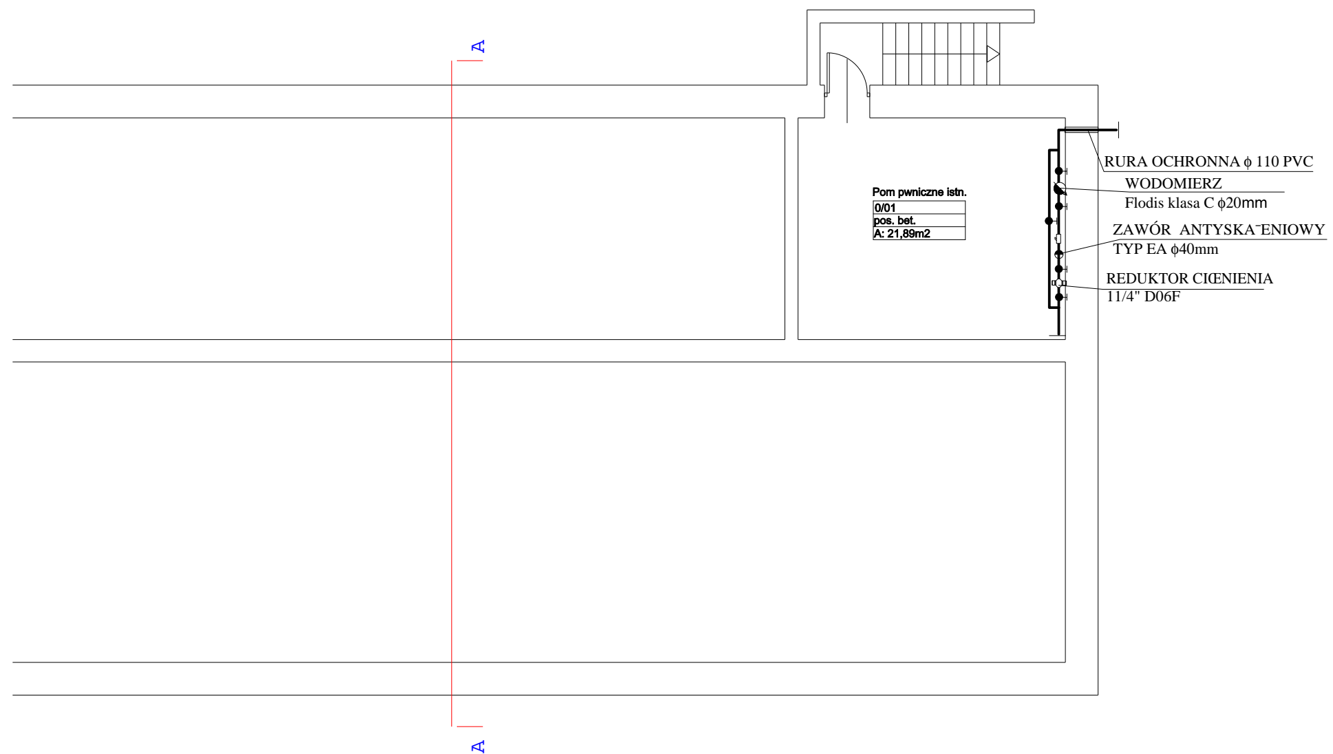
RZUT PIWNIC 1:100
